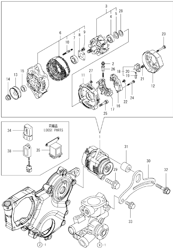
0CW10-M34200 3TNM68-GGE/HGE Fig.17. (15A)GENERATOR
