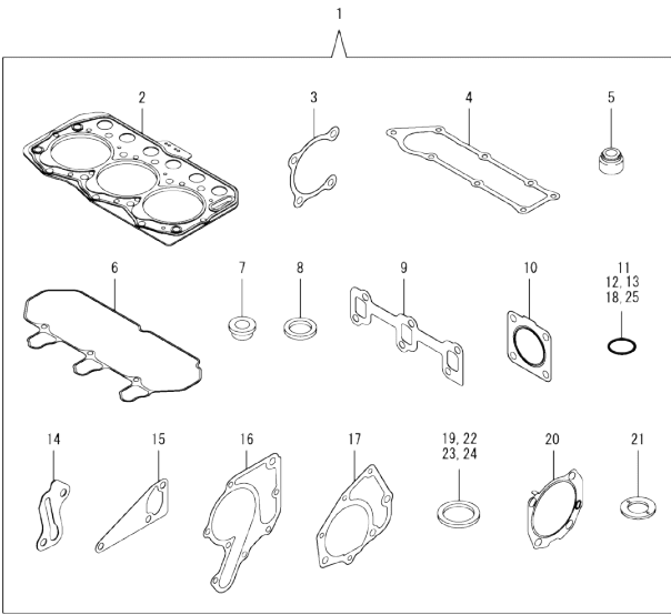
Fig.16. GASKET SET
